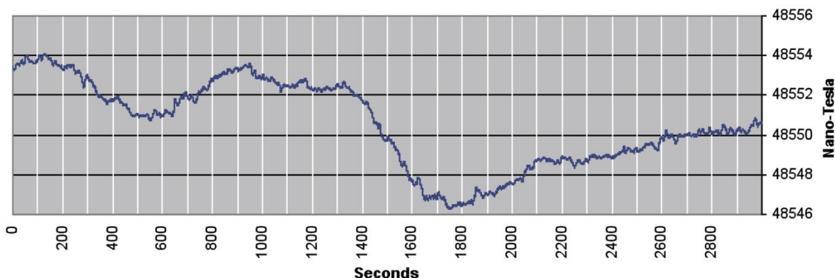
Запись вариаций магнитного поля, измеренная с помощью G-862RBS при частоте 10 Гц.
