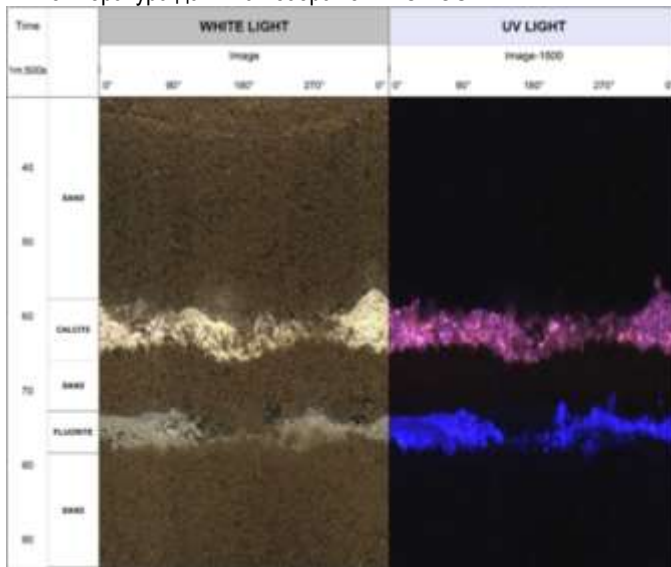
Белый свет в сравнении с ультрафиолетовым – флуоресценция минералов в песчанике (кальцит окрашен в розовый цвет, а плавиковый шпат – в синий)
